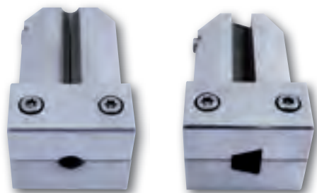
Formnest für Rundriemen
