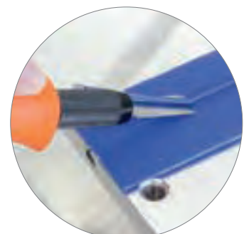
Einfaches Entfernen des Schweißwulstes mit dem mitgelieferten Werkzeug
