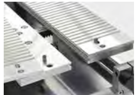
Arretierstifte sorgen für die richtige Positionierung der Adapterplatten auf dem Fügetisch.
